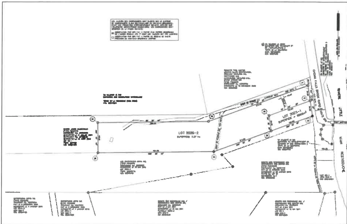
Figure 4: Plan de subdivision tentatif
