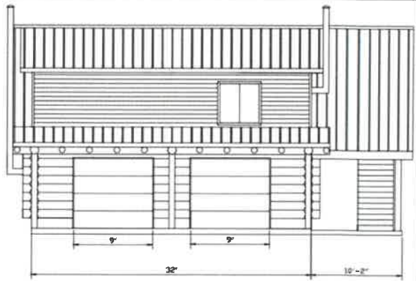
Elevation 1
